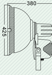
SD7a-G-2 (85W)
